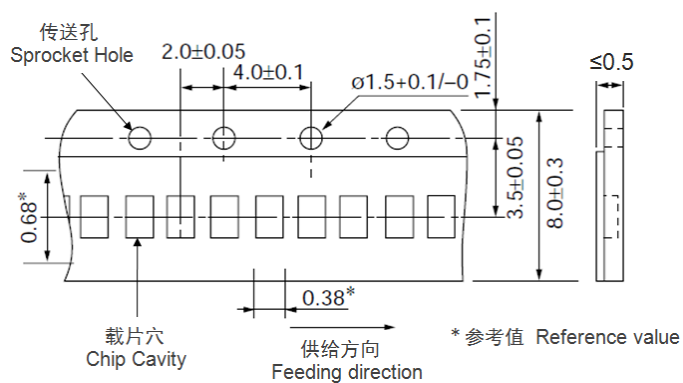
0201 系列 0201 series
