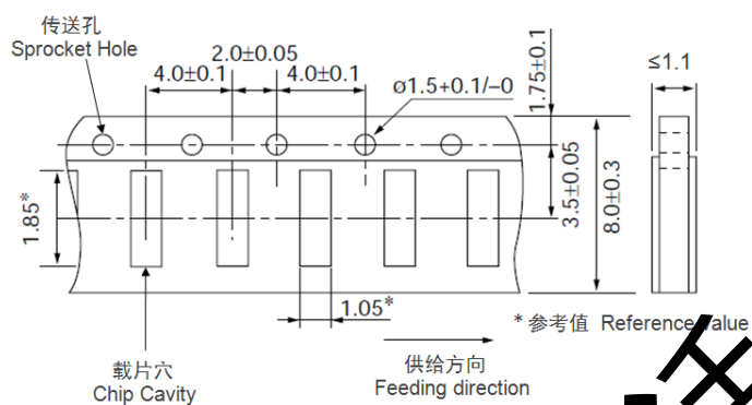
0603 系列 0603 series
